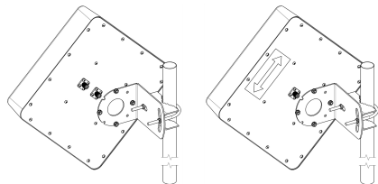
Рисунок 3 – X-поляризация
