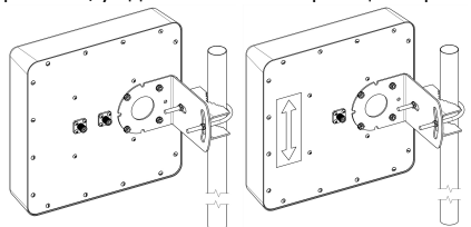
Рисунок 2 – Монтаж антенны на мачте
